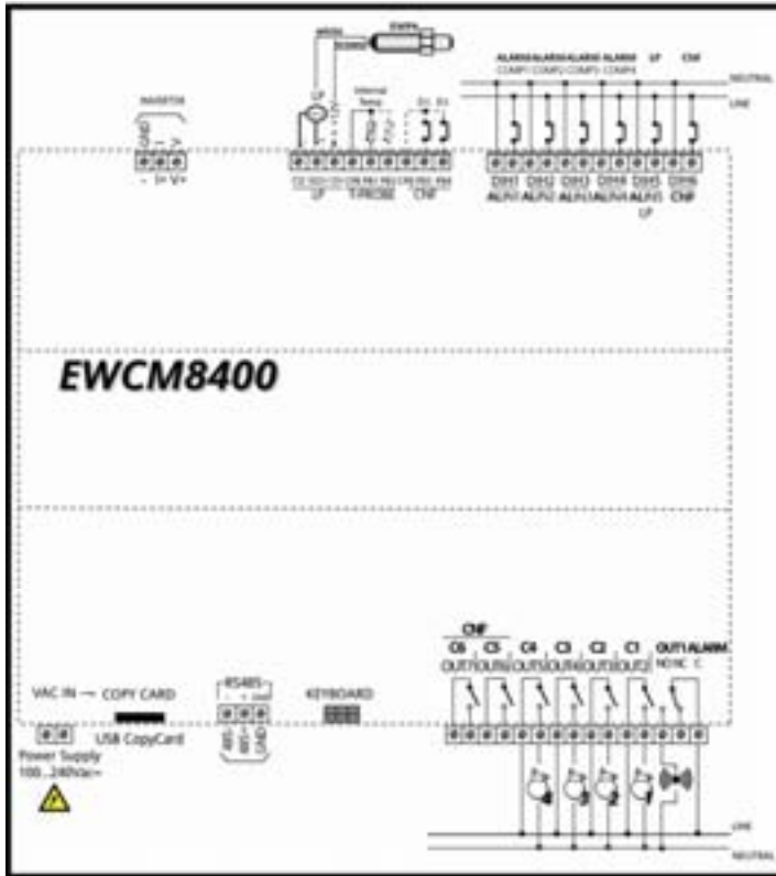
4 ступени компрессора и/или инвертер
