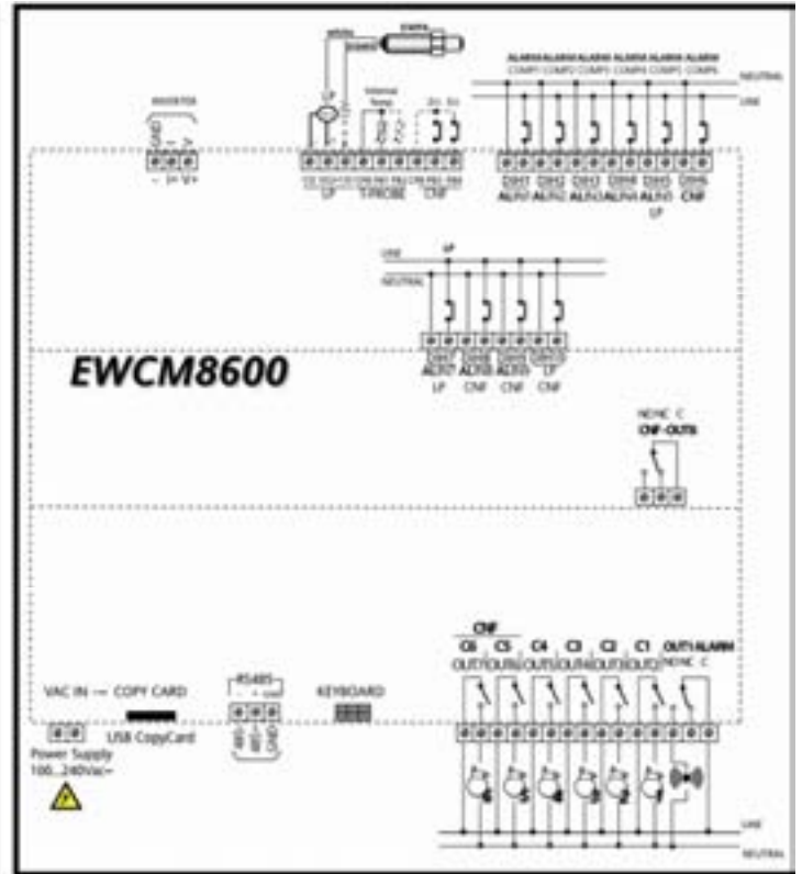
6 ступеней компрессора и/или инвертер
