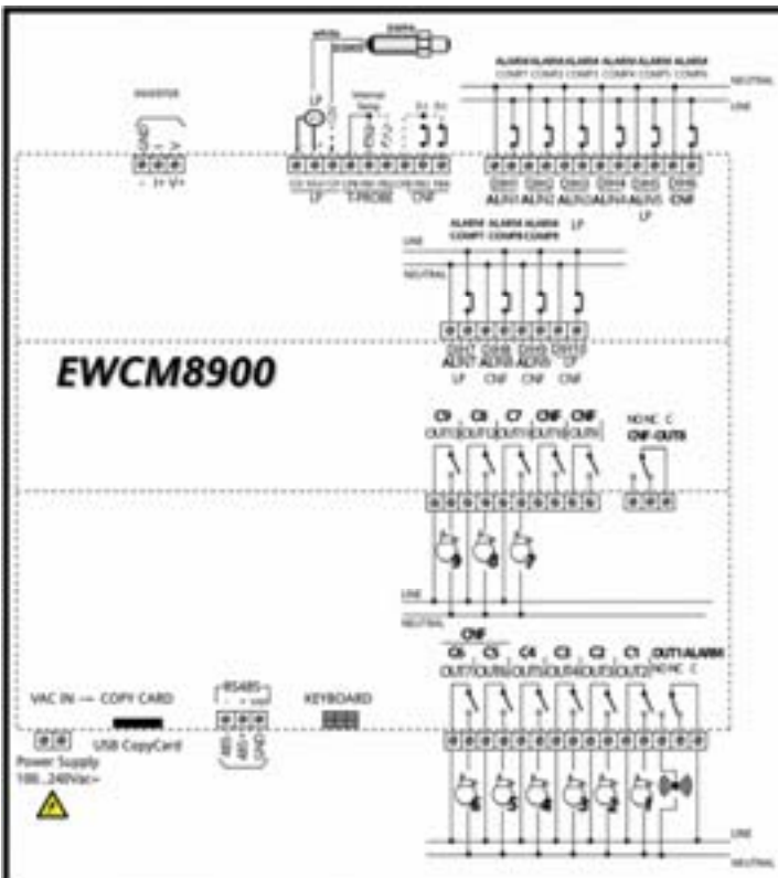
9 ступеней компрессора и/или инвертер
